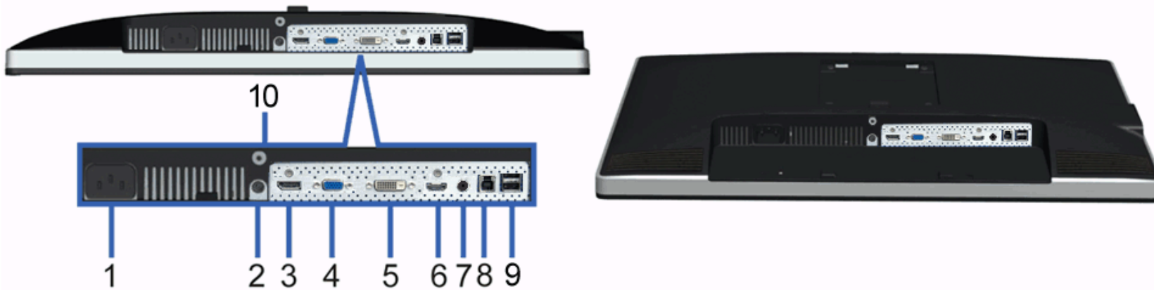
Tampilan Bawah
